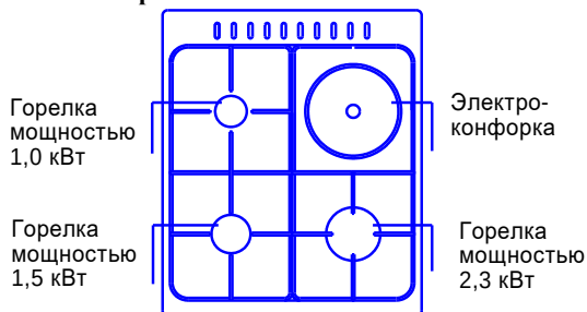
Рис. 14. Верхняя панель плит CGE-531 ecWh
