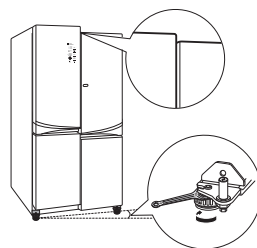
3 Выравнивание положения холодильника и дверцы
