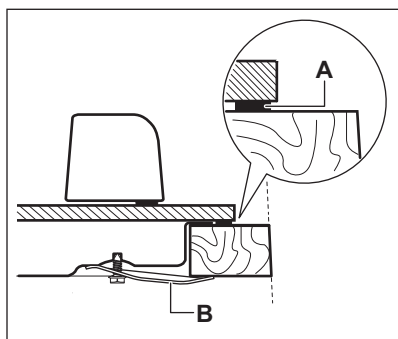
А) ущільнювач, що постачається В) скоби, що постачаються
