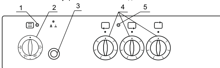
Панель управления плиты модели 5003.17э
