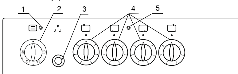
Панель управления плит моделей 5004.13э, 5004.14э
