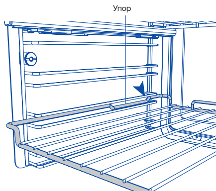
Установка полки на держатели
